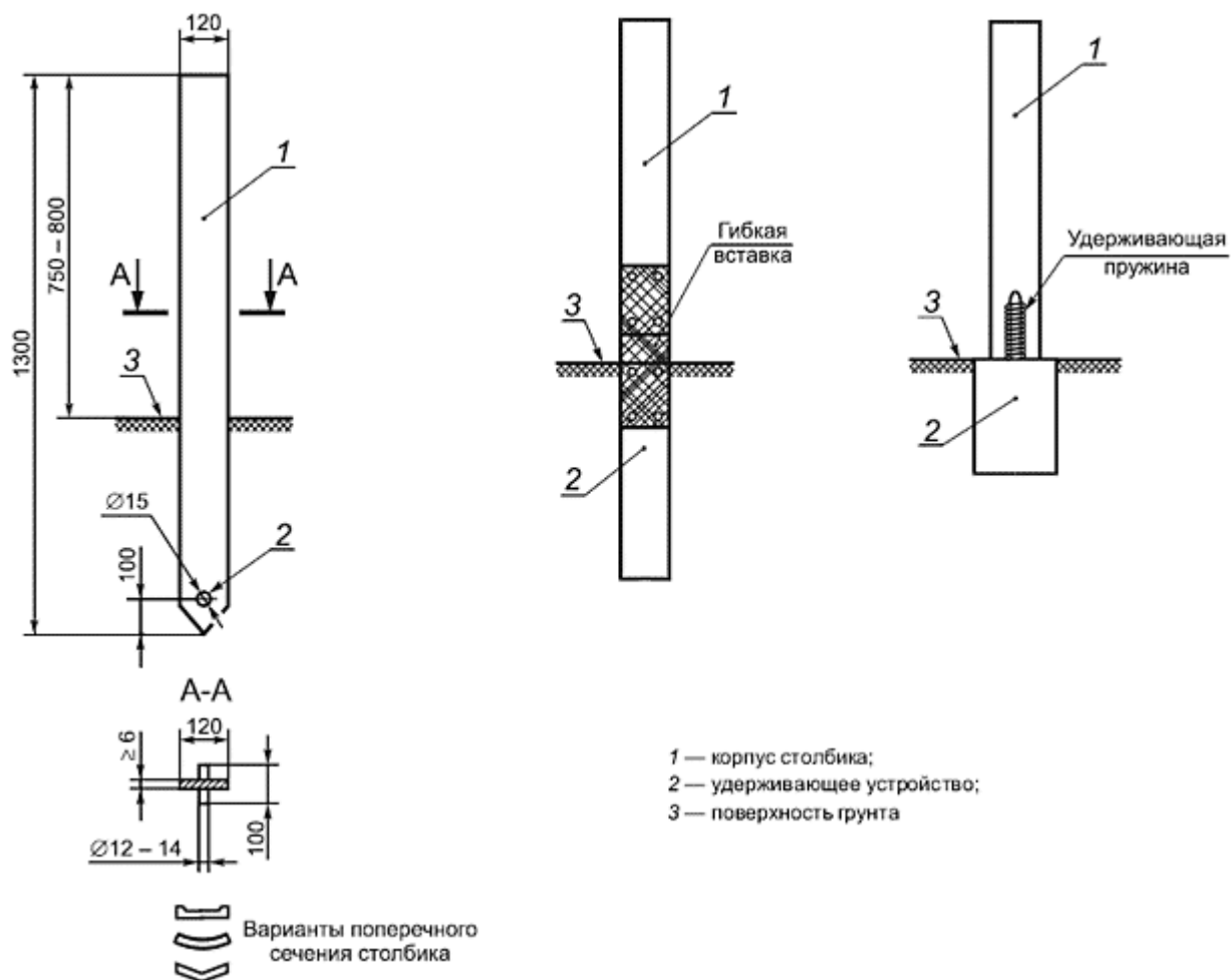
Рисунок 5 - Сигнальный столбик типа С2
